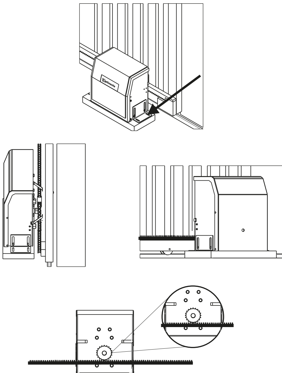
Figura 03: Fixar a cremalheira no portão, com um ponto de solda, observando que a engrenagem se encaixa na cremalheira, para que ocorra a movimentação do portão no momento que o movimentador for acionado.
